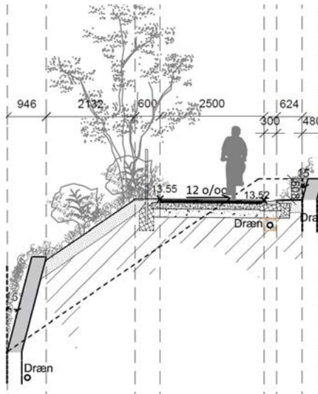
Tværsnit af en af de to cykelramper, der skal anlægges parallelt med Langesøstien ind i skrånten. Tegning: VandcenterSyd
