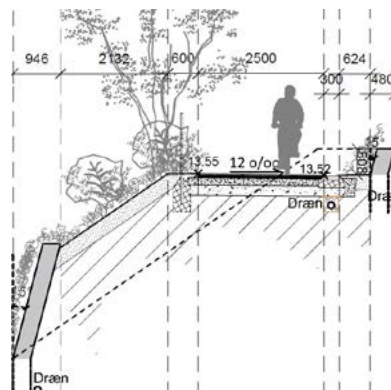
Tværsnit af den ene cykelrampe med støttemur ned mod Langesøstien (tv.). Illustration: VandcenterSyd
